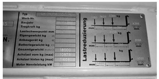
3 An jedem Stapler muss ein gut lesbares Tragkraft-Diagramm angebracht sein.
